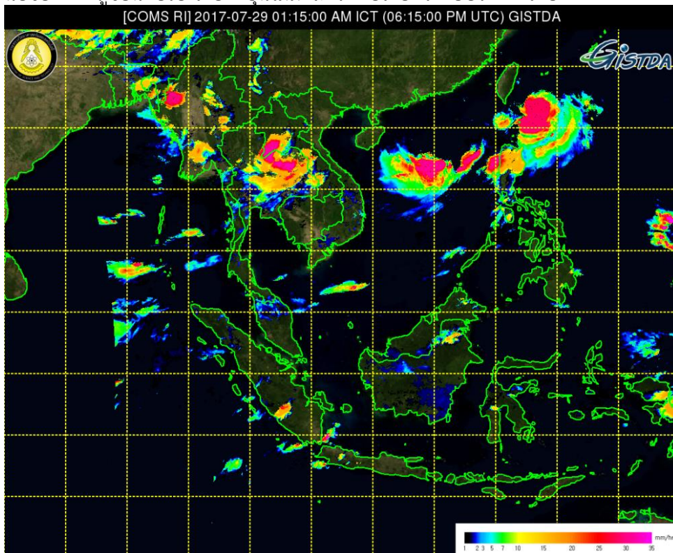
ภาพที่ 1 ข้อมูลจากดาวเทียม COMS แสดงสภาพอากาศ ณ วันที่ 29 กรกฎาคม 2560 เวลา 06.15น.
