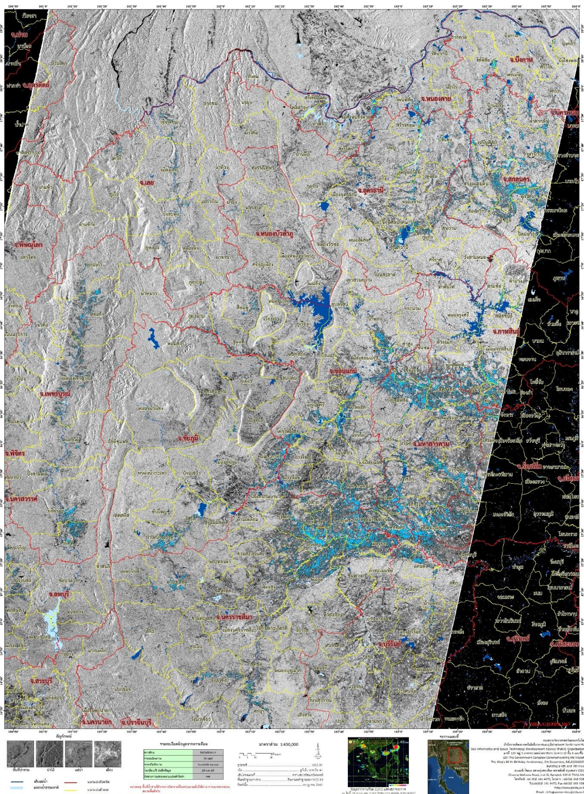
ภาพที่ 1 พื้นที่น้ำท่วม (สีฟ้า) จากการวิเคราะห์ข้อมูลจากดาวเทียม บันทึกภาพ Radarsat-2 วันที่ 29 กรกฎาคม 2560 เวลา 06.06 น.บริเวณบางส่วนของภาคตะวันออกเฉียงเหนือ
