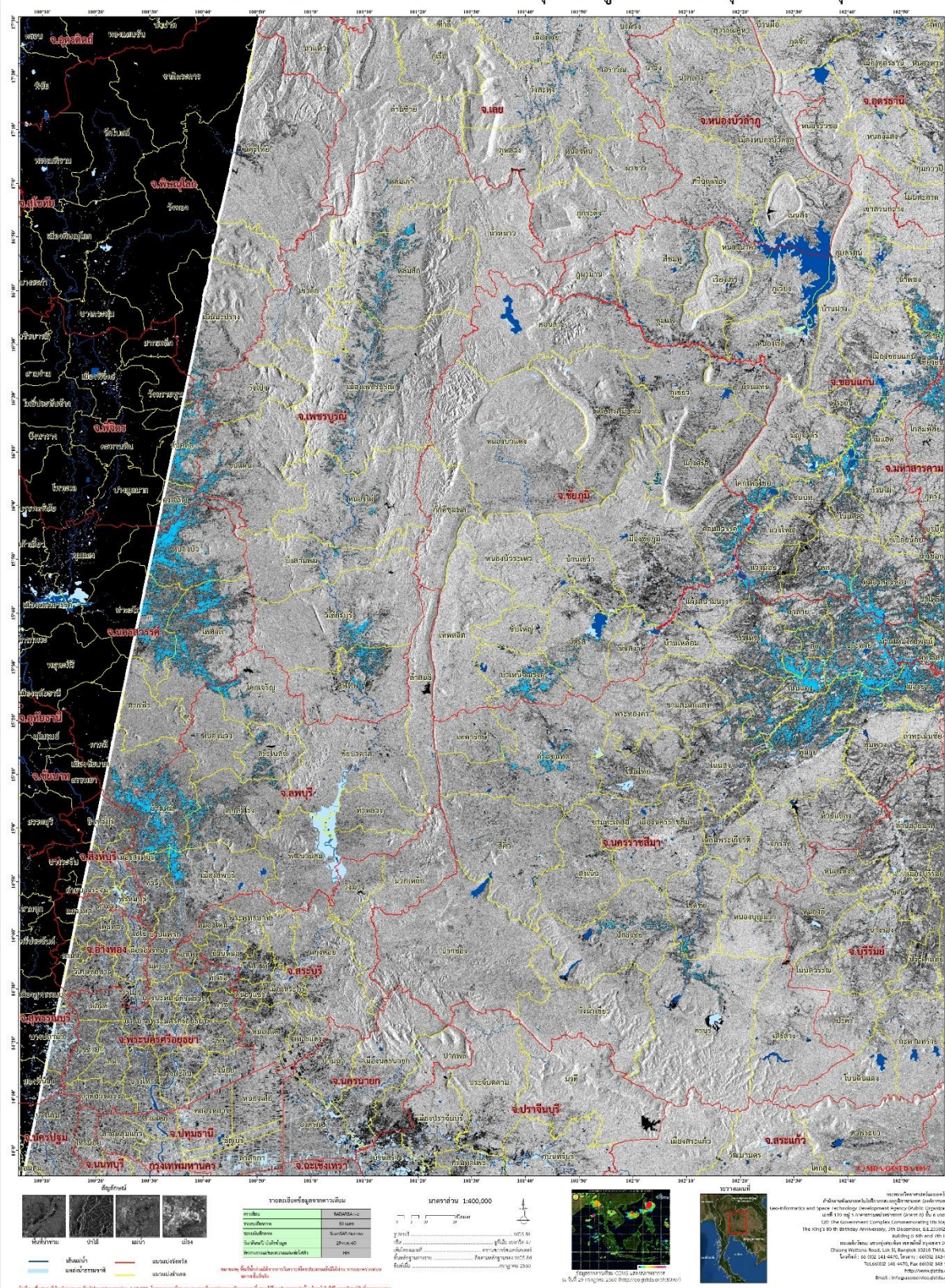
ภาพที่ 2 พื้นที่น่าท่วม (สีฟ้า) จากการวิเคราะห์ข้อมูลจากดาวเทียม บันทึกภาพ Radarsat-2
